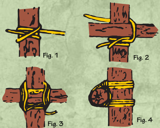
Amarre cuadrado
