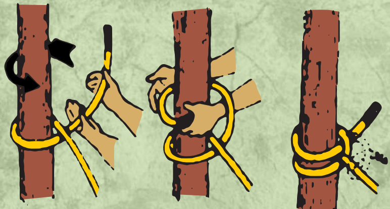
Nudo ballestrinque
